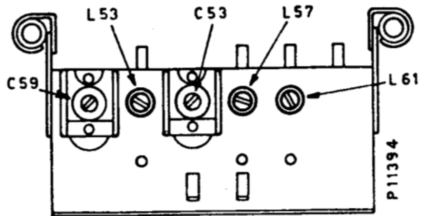
Gruppo R.F. Mod. di amp. - Vista posteriore
